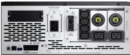
[ SMX3000HV ]
